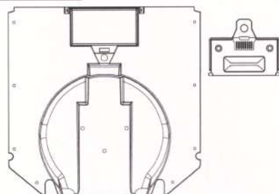
P7171A Bucket Plate 凹凸板 2pc
